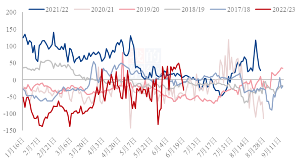
图 13 淀粉 9/1 价差
