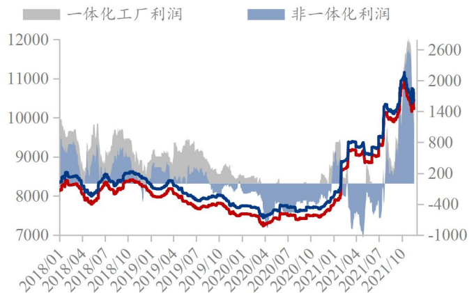
201冷轧成本及即期利润（元/吨）
