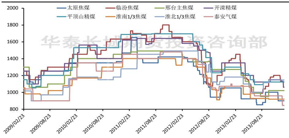
图 15: 我国部分主产地炼焦煤价格 (元/吨) (2009.2-2014.1)
